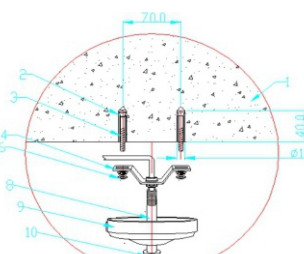
LED教室灯安装示意图
