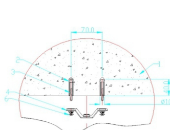
LED教室灯安装示意图
